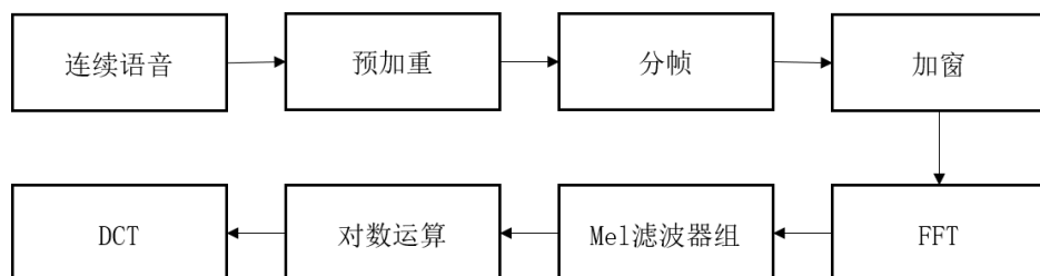
图 3-5: MFCC 特征提取流程
